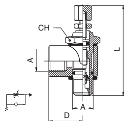
REGOLATORE UNIDIREZIONALE PER VALVOLA REGOLAZIONE A CACCIIVITE UNI-DIRECTIONAL FLOW REGULATOR FOR VALVE SCREWDRIVER REGULATION
