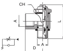
REGOLATORE UNIDIREZIONALE PER VALVOLA REGOLAZIONE MANUALE UNI-DIRECTIONAL FLOW REGULATOR FOR VALVE MANUAL REGULATION
