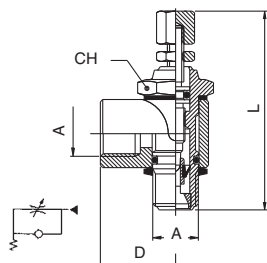
REGOLATORE UNIDIREZIONALE PER VALVOLA REGOLAZIONE MANUALE UNI-DIRECTIONAL FLOW REGULATOR FOR VALVE MANUAL REGULATION
