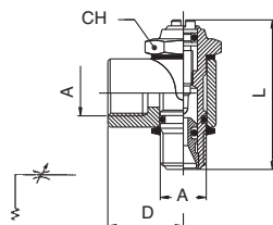
REGOLATORE BIDIREZIONALE REGOLAZIONE MANUALE BI-DIRECTIONAL FLOW REGULATOR MANUAL REGULATION
